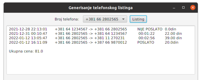
Slika 4: Generisanje listinga
